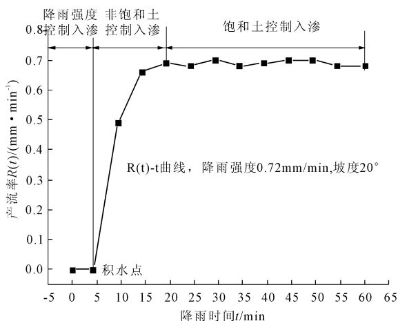
图 4 坡面产流率随降雨时间变化规律曲线
